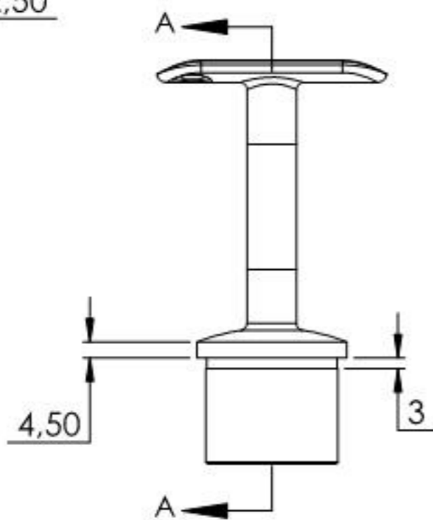
SCHNITT A-A
