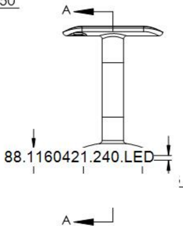
SCHNITT A-A
