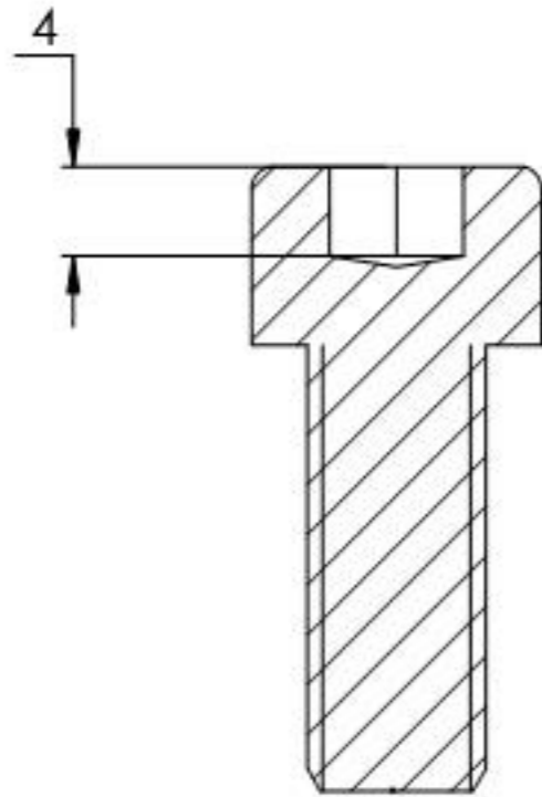
SCHNITT A-A
