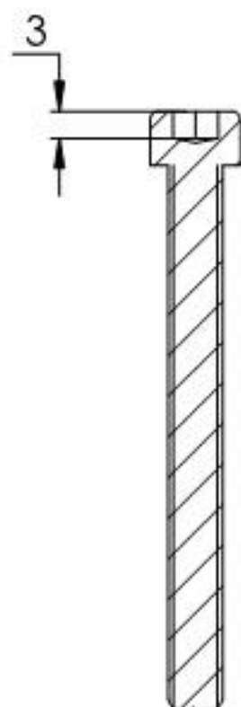
SCHNITT A-A
