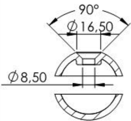
SCHNITT C-C
