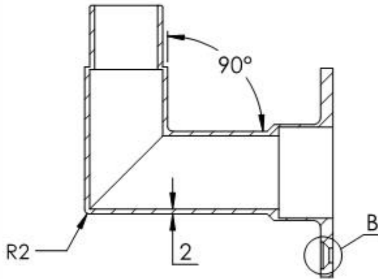
SCHNITT A-A
