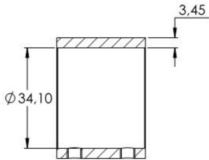
SCHNITT B-B
