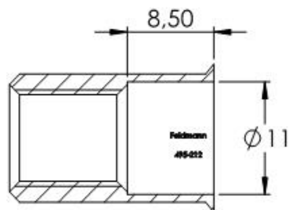
SCHNITT A-A
