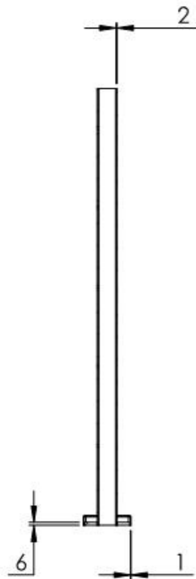
SCHNITT A-A
