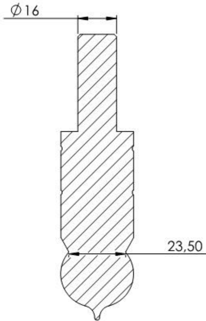
SCHNITT B-B
