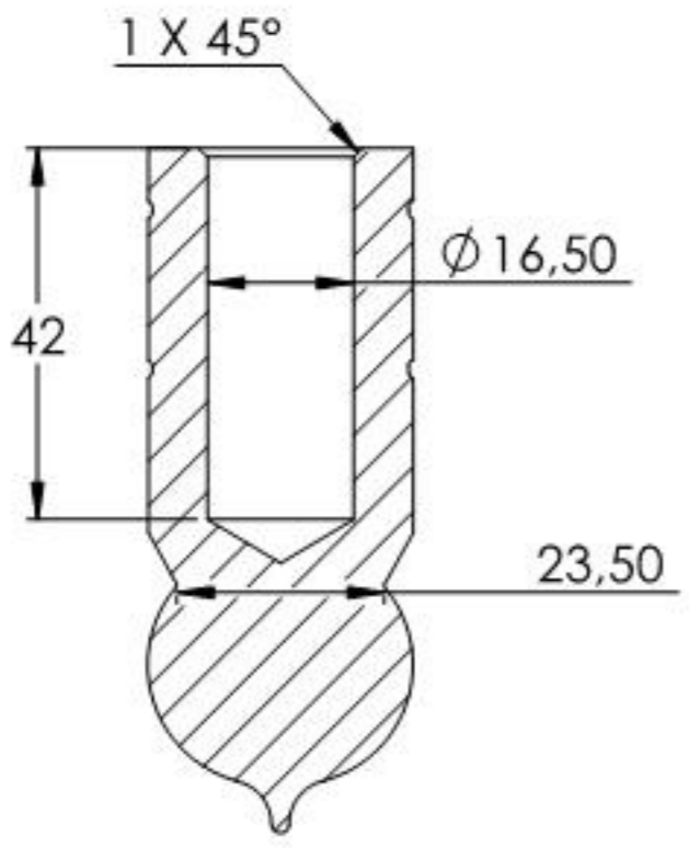
SCHNITT C-C
