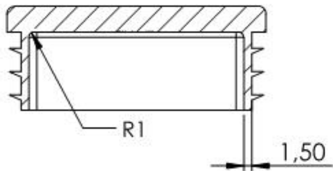
SCHNITT A-A
