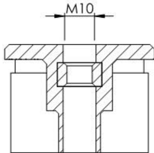
SCHNITT A-A
