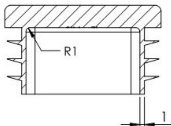
SCHNITT A-A
