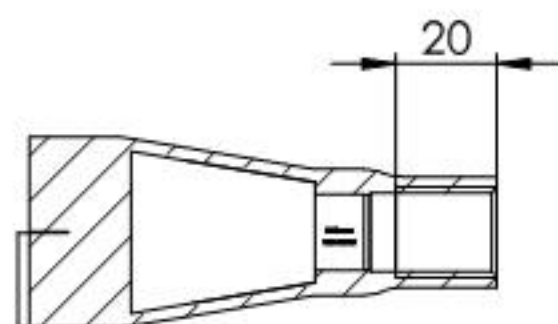
SCHNITT A-A
