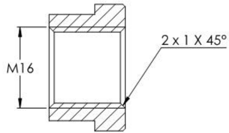
SCHNITT A-A
