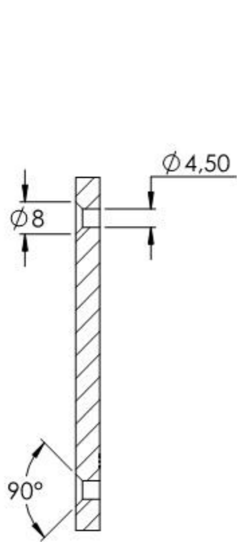
SCHNITT A-A
