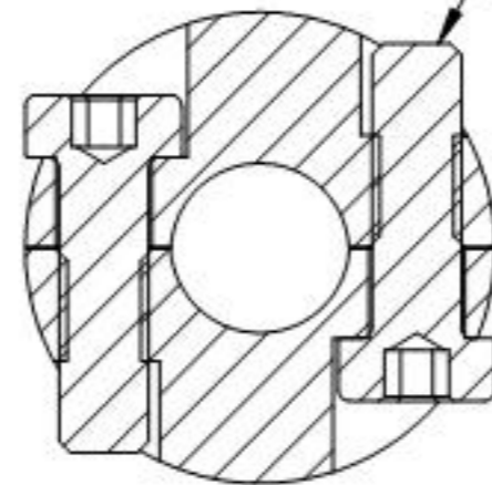
SCHNITT A-A
