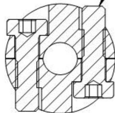
SCHNITT A-A
