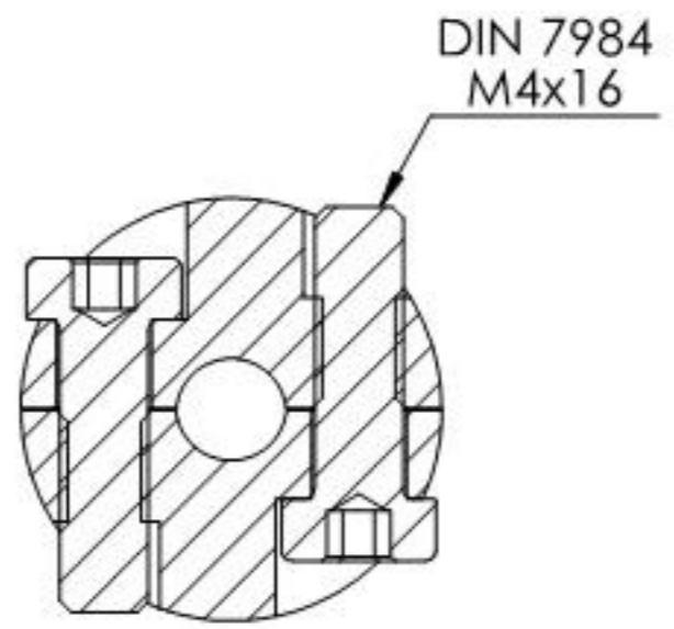
SCHNITT A-A
