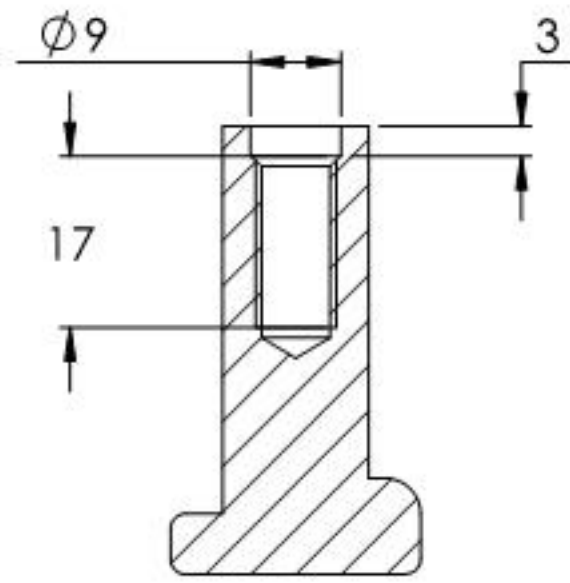
SCHNITT B-B
