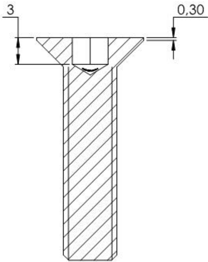
SCHNITT A-A
