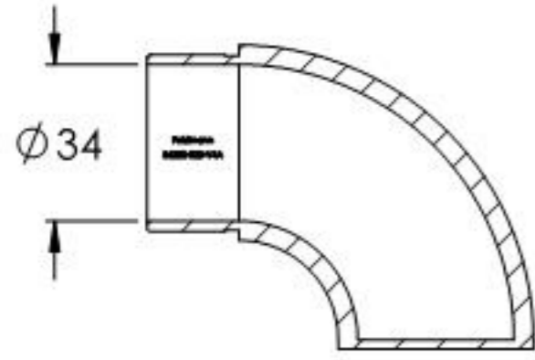
SCHNITT A-A
