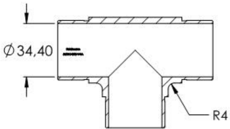
SCHNITT A-A
