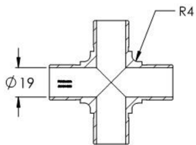
SCHNITT A-A
