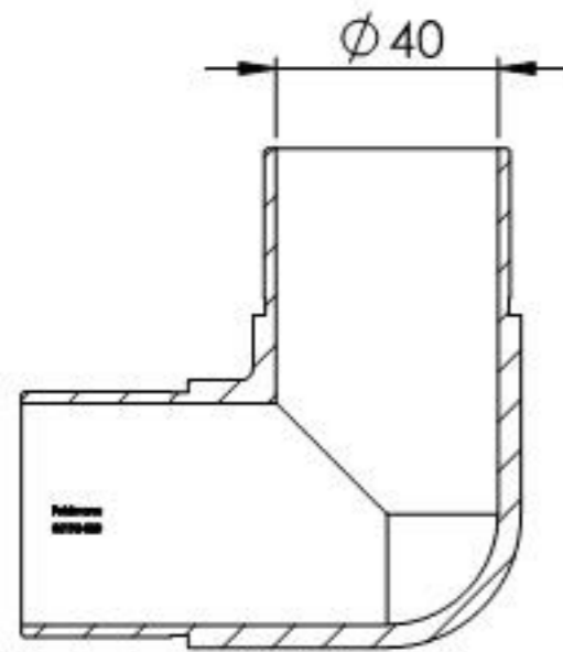
SCHNITT A-A
