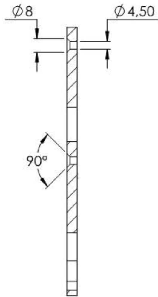
SCHNITT A-A
