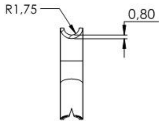
SCHNITT A-A
