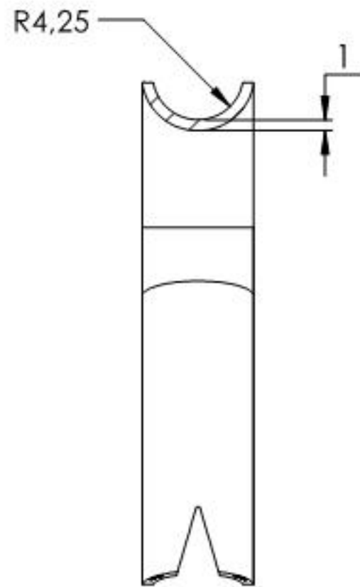
SCHNITT A-A
