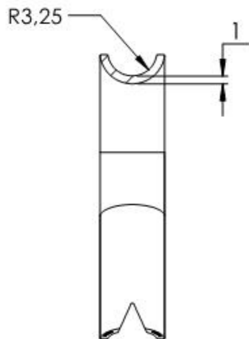
SCHNITT A-A
