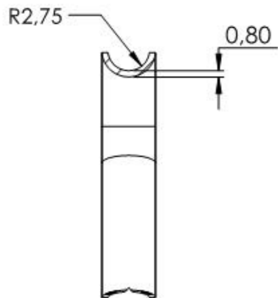
SCHNITT A-A
