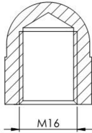
SCHNITT A-A
