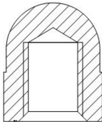
M6 SCHNITT A-A
