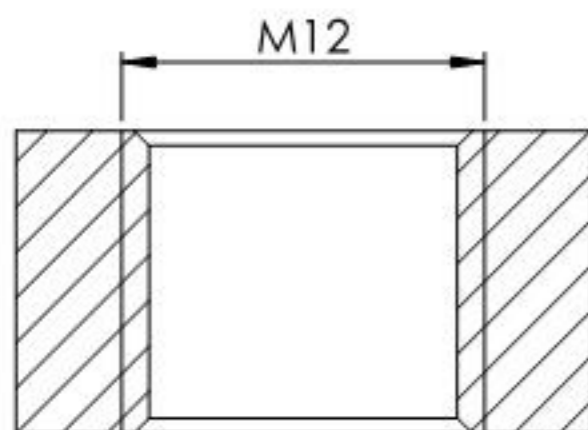
SCHNITT A-A
