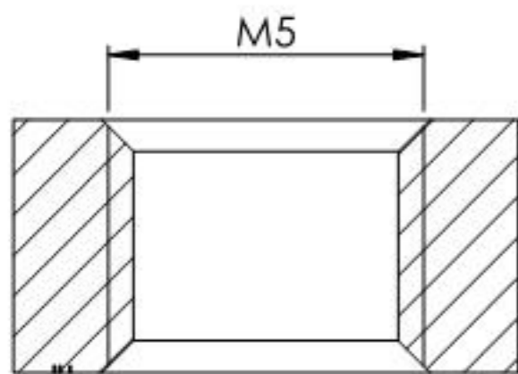
SCHNITT A-A
