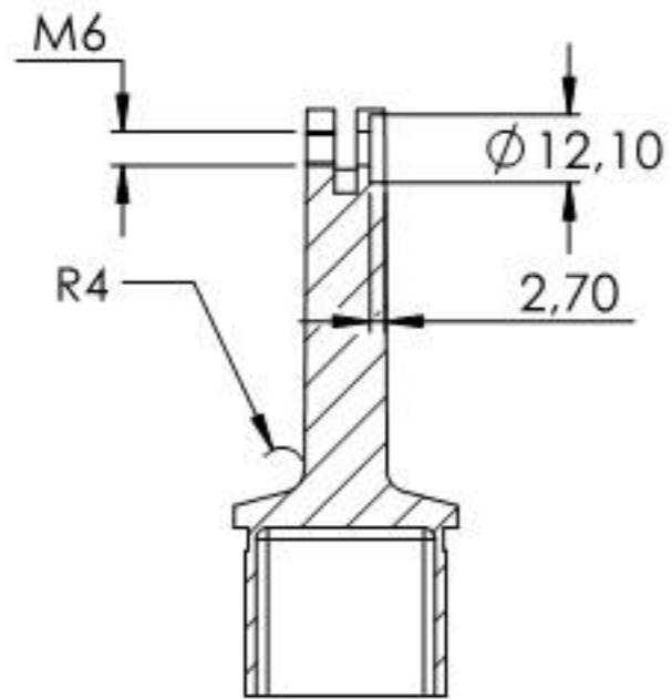
SCHNITT A-A
