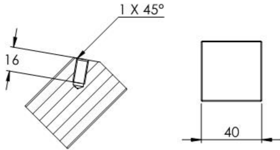
SCHNITT A-A
