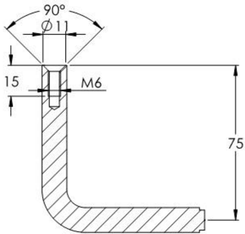
SCHNITT B-B
