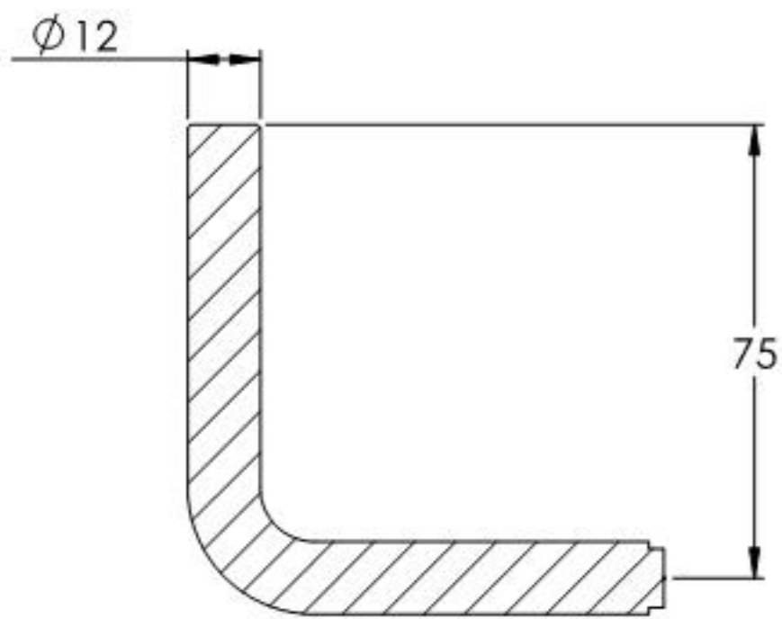
SCHNITT B-B
