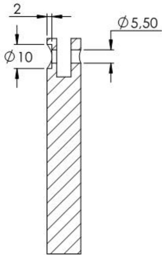
SCHNITT C-C
