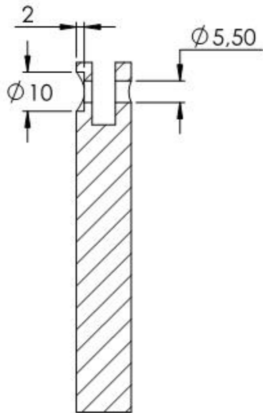
SCHNITT C-C
