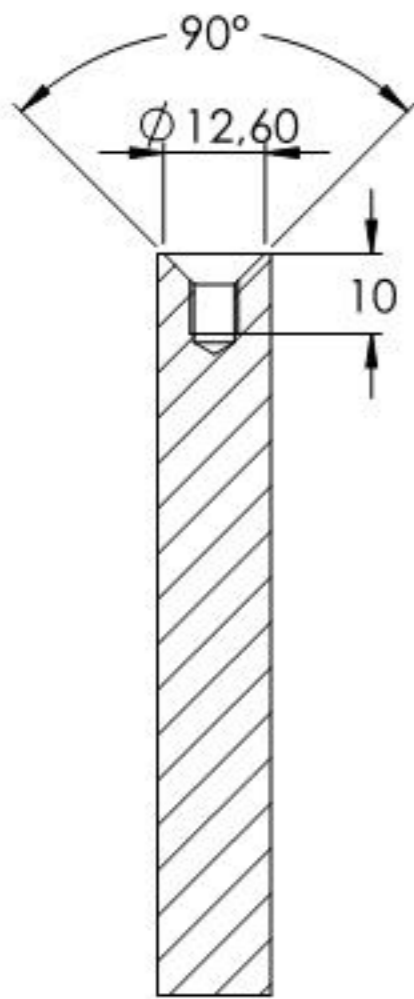
SCHNITT C-C
