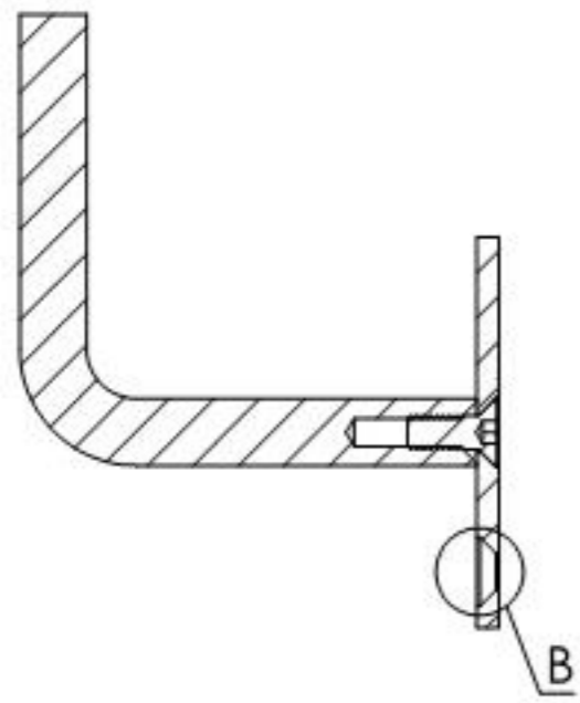
SCHNITT A-A
