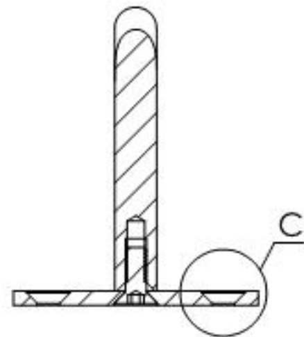
SCHNITT B-B
