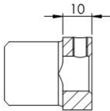
SCHNITT D-D
