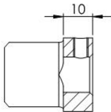
SCHNITT D-D
