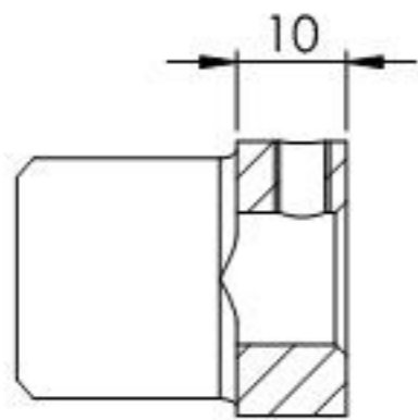
SCHNITT D-D
