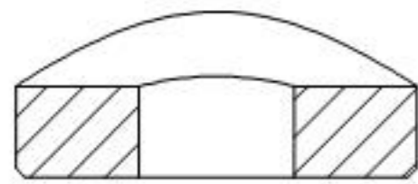
SCHNITT A-A
